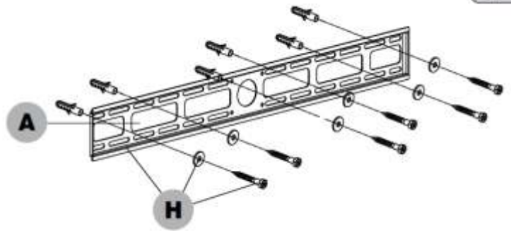
Installation auf Wänden als Mauerwerk
