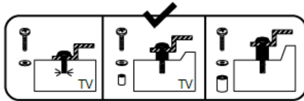
Installation auf Wänden als Mauerwerk
