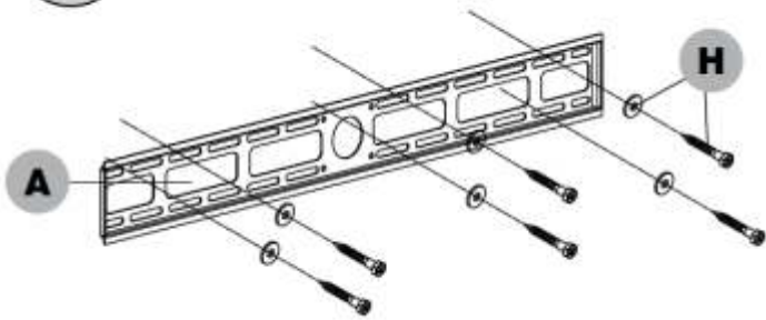
Installation auf Wänden mit Holzrahmen
